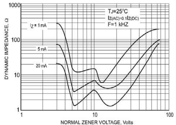
FIG. 2-EFFECT OF ZENER VOLTAGE ON ZENER IMPEDANCE
