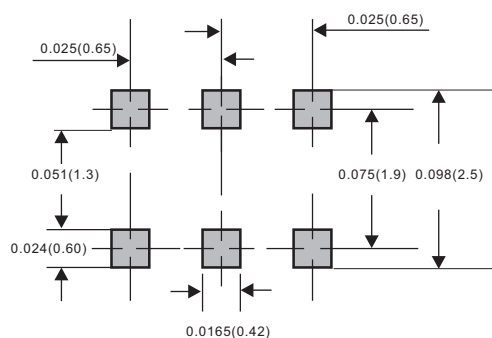
SOT-363
