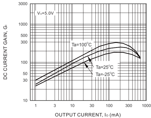
G_i - I_o
