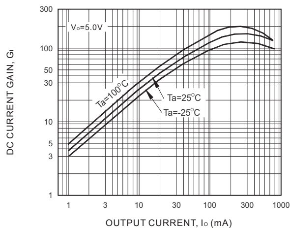
G_i - I_o
